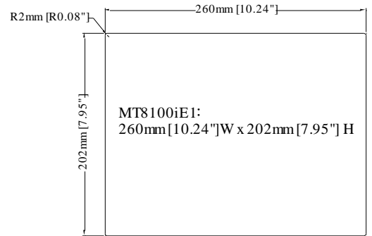
Cutout Dimensions
